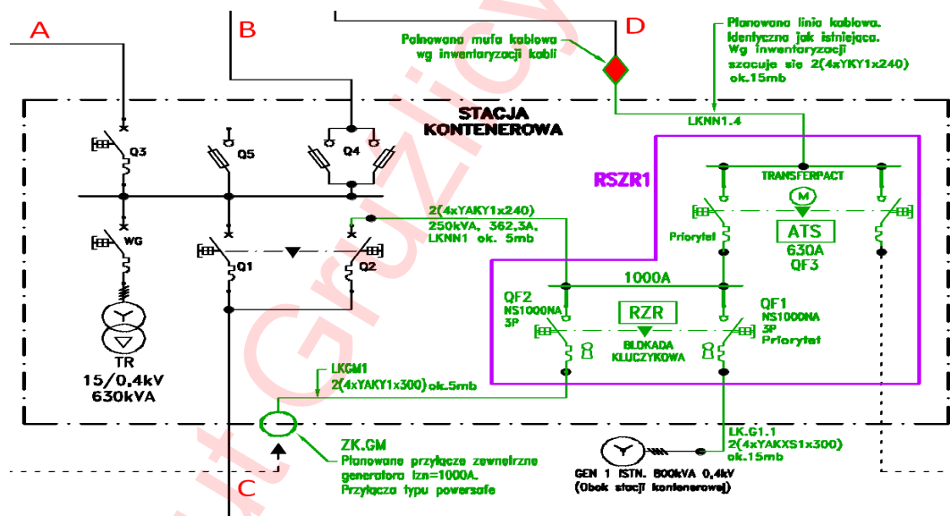
Rys. 2 Planowany schemat przebudowy zasilania Instytutu
